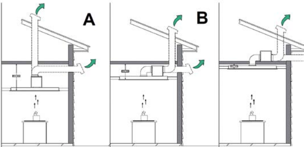
Einbauvarianten CARINA
